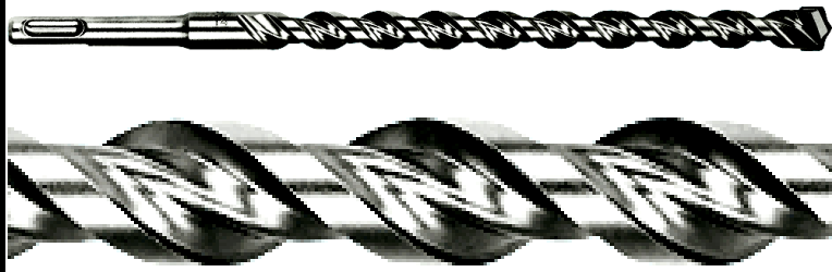
Foret béton reca Ultra (sans revêtement MolySpeed) Référence : 0651 0.. ..0 De 16mm à 26 mm (jusqu'à 450mm)
